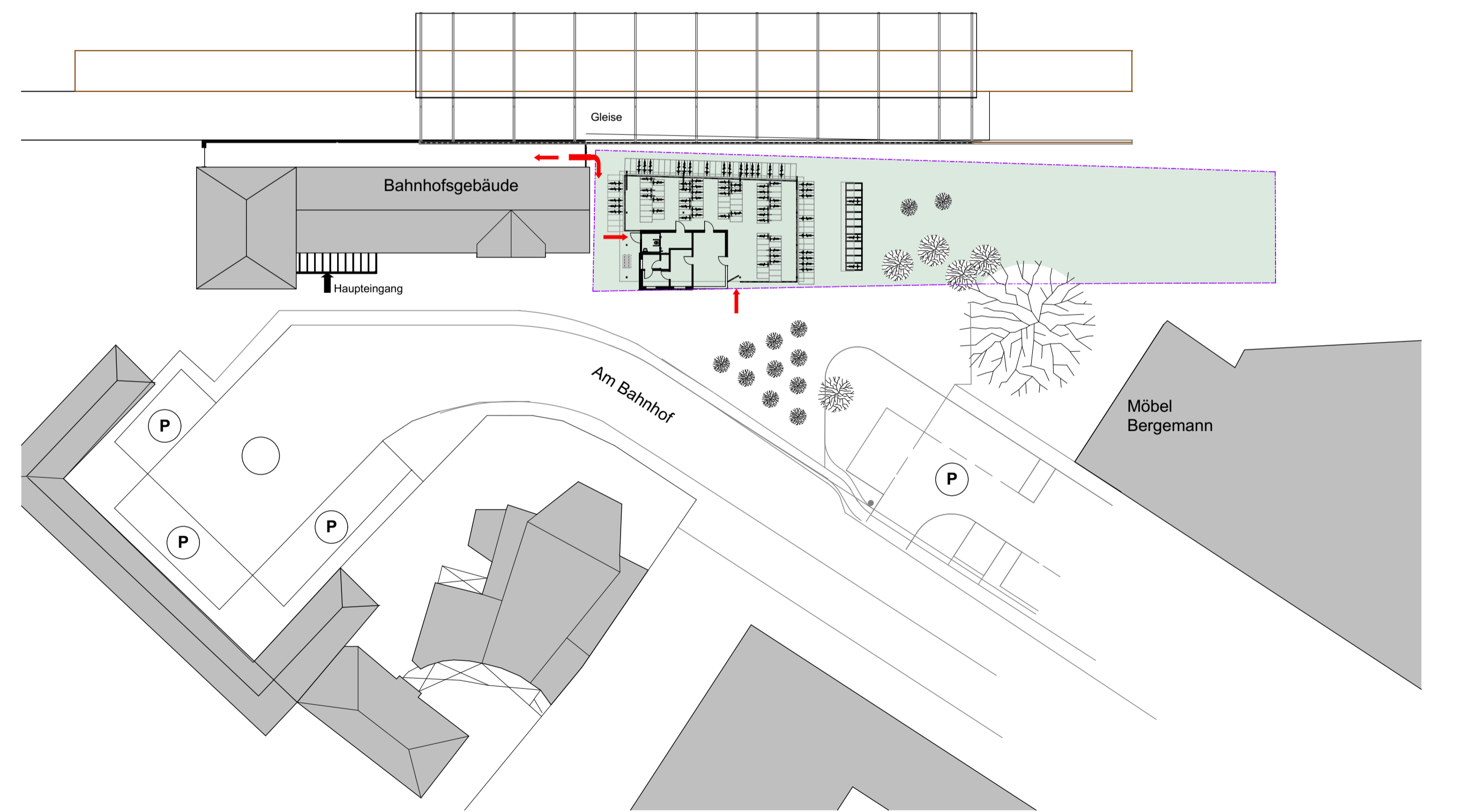
LAGEPLAN 1:500
